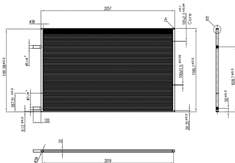
3- کندانسور آلومینیومی مایکروچنل D2000
