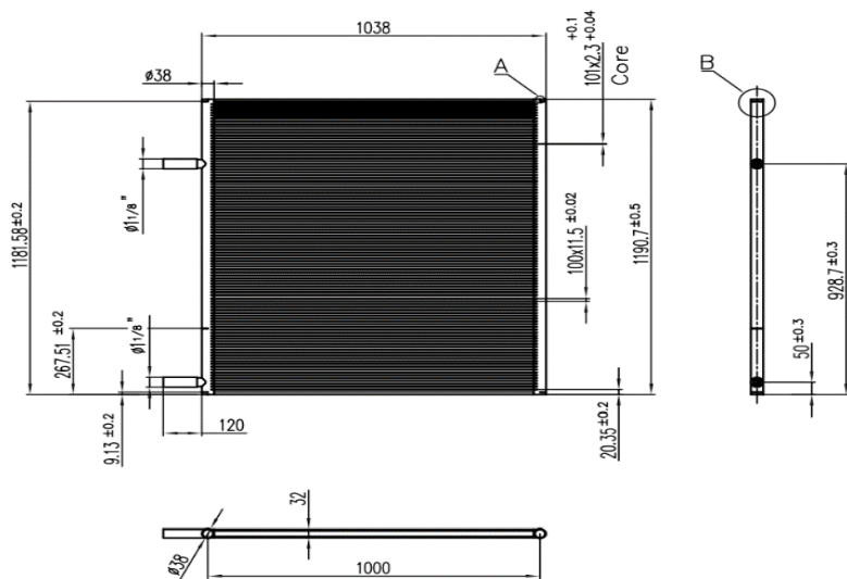
2- کندانسور آلومینیومی مایکروچنل D1000
